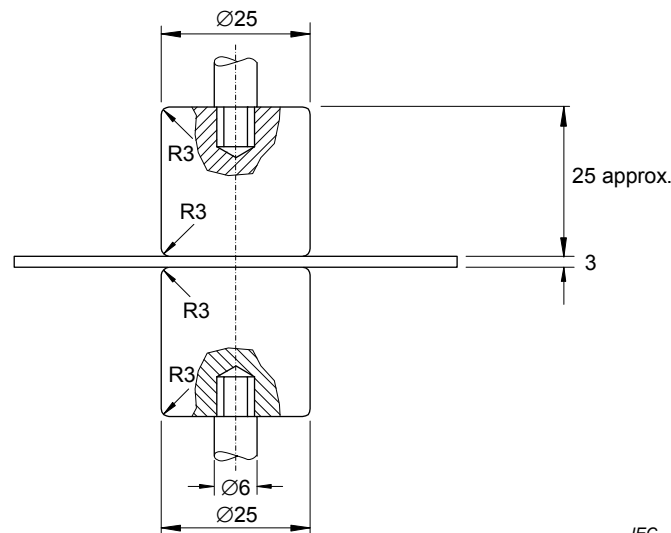
Figure 1b – Électrodes de même diamètre
