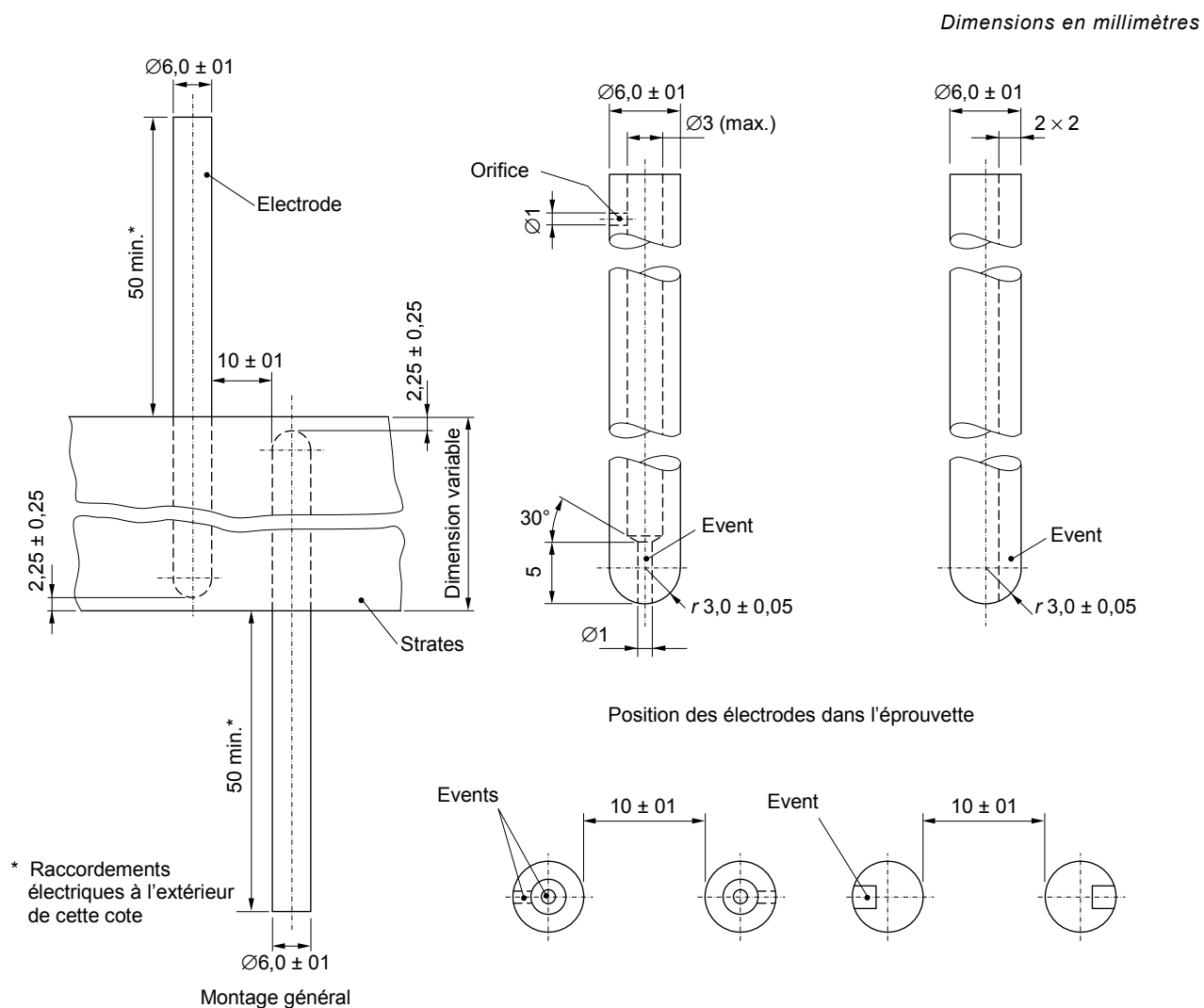
Figure 8 – Dispositif pour les essais effectués parallèlement aux strates avec électrodes cylindriques parallèles (planches > 15 mm d'épaisseur) (voir 5.3.4)
