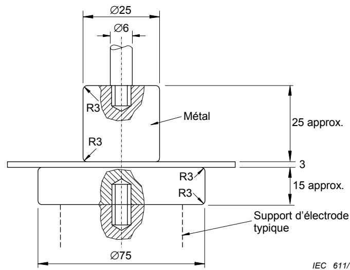
Figure 1a – Électrodes de dimensions inégales
